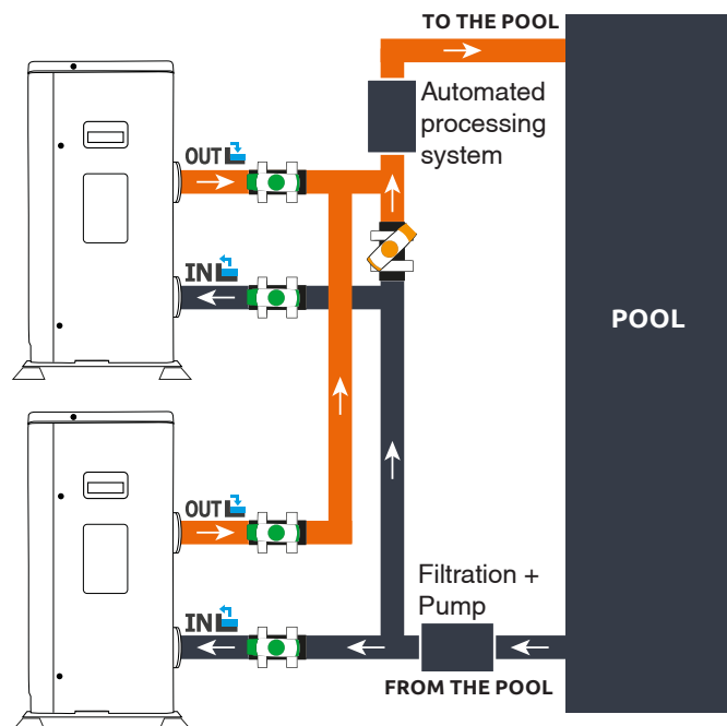
Serie assembly
