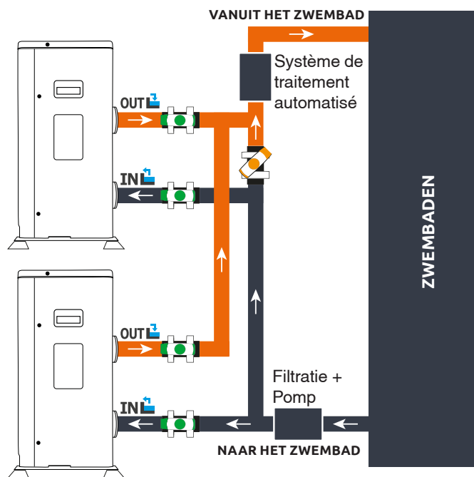
Serie montage
