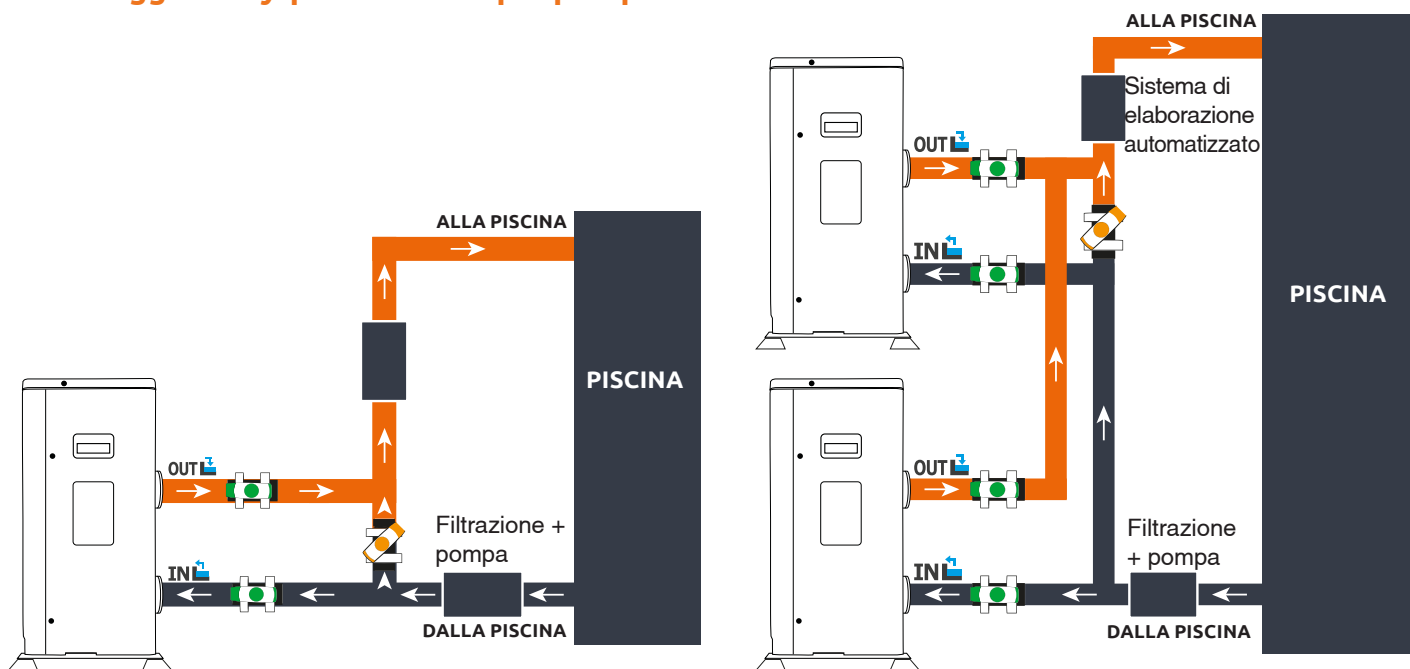
Montaggio semplice
