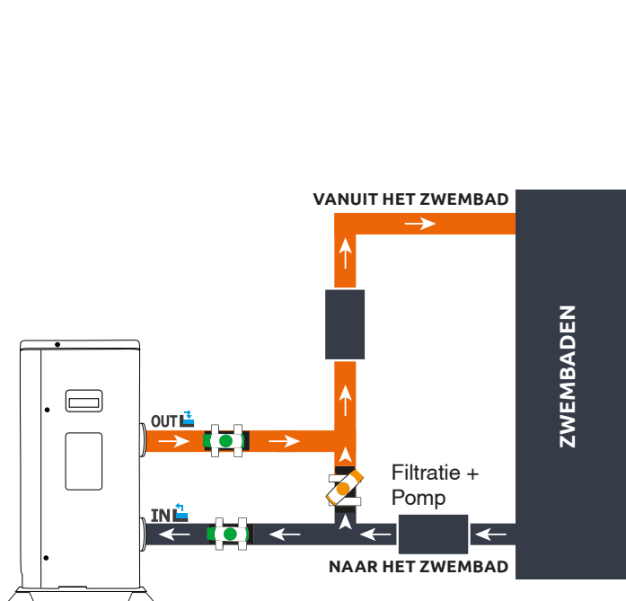
Eenvoudige montage
