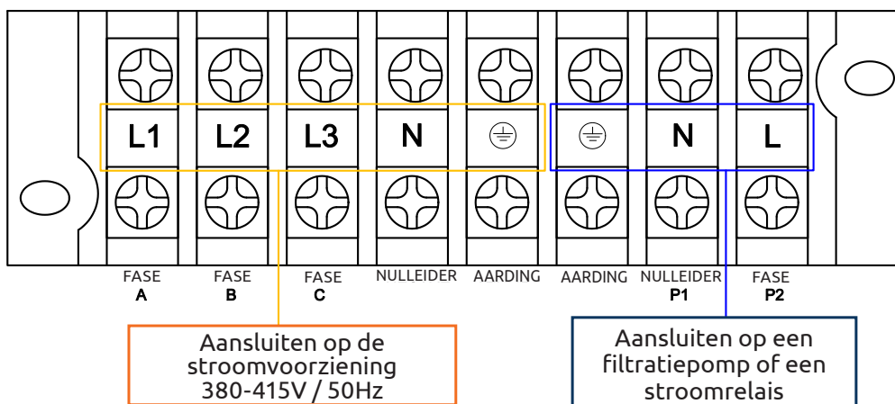
Driefasemodel
